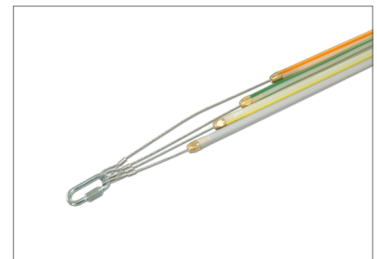
Beispiel Ziehkopf
