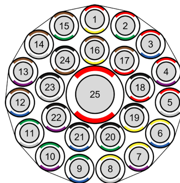
Beispiel: HexaSpeed 24×7×1,5 + 1×14×2,0
